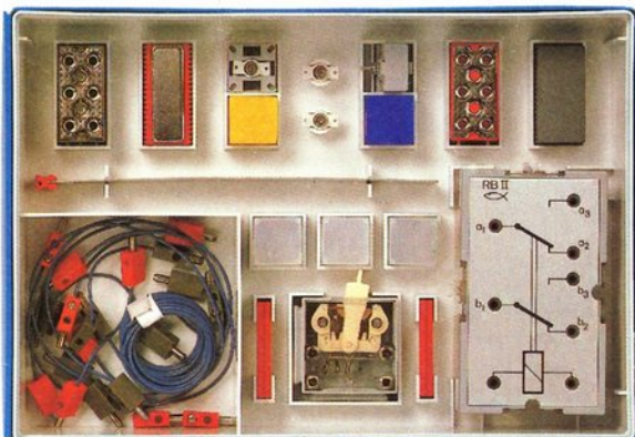
em 3 elektromechanica relais, poolwisselaar bimetaal, Art.nr. 30232
