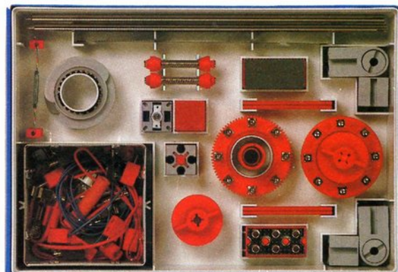
em 2 elektromechanica etappenschakelaar, magneet stuuronderdelen, Art.nr. 30231
